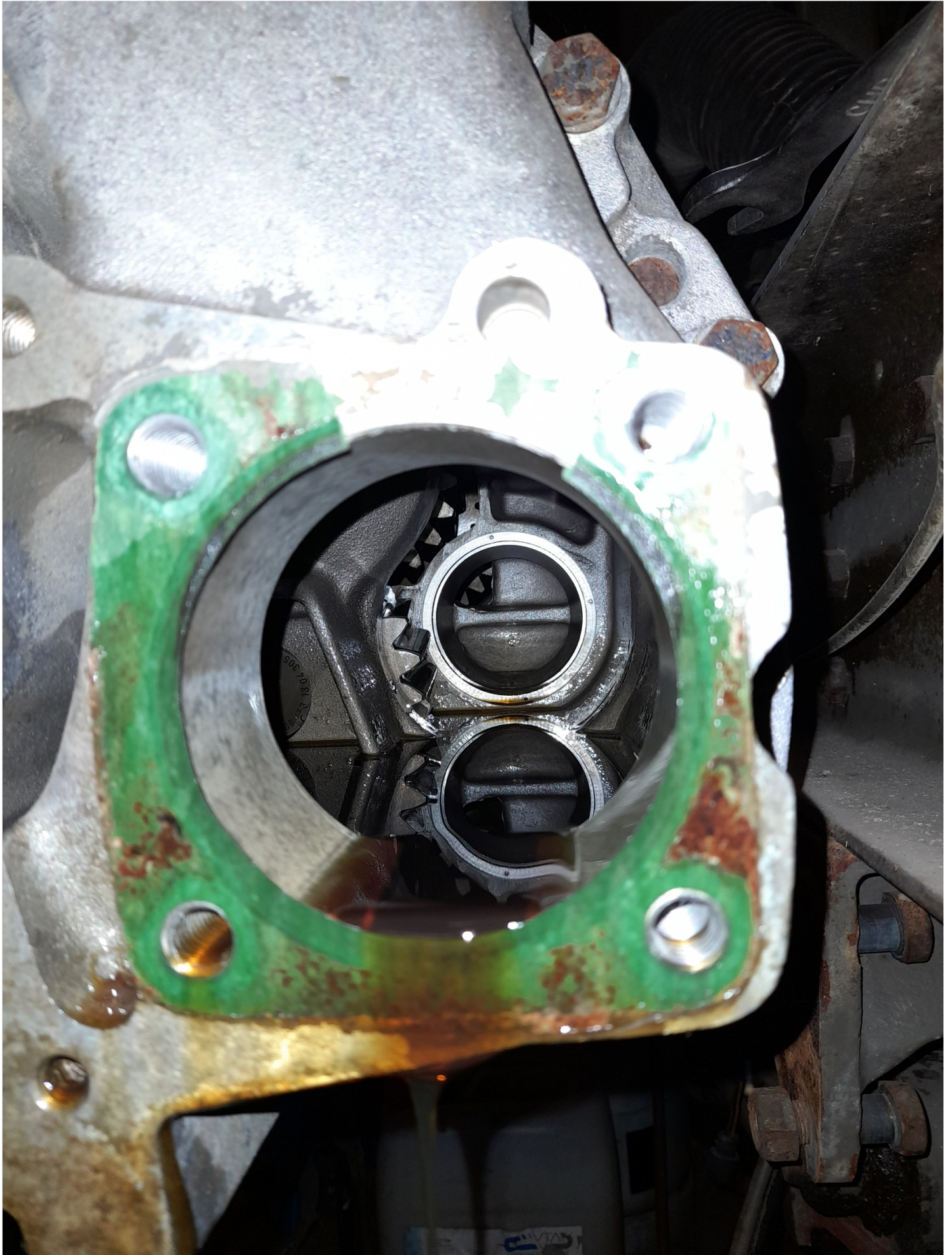
Blick ins Innere des Getriebes
